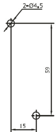
安装孔尺寸
