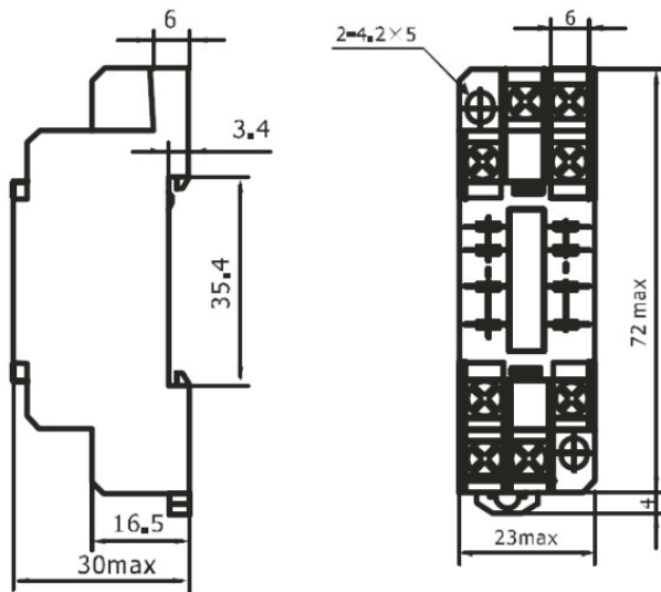
外形图
